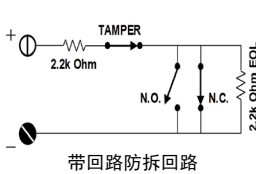
带回路防拆回路
